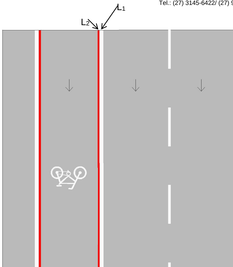
Figura 2: Marcação de ciclovia quando não houver possibilidade da superfície ser totalmente vermelha
