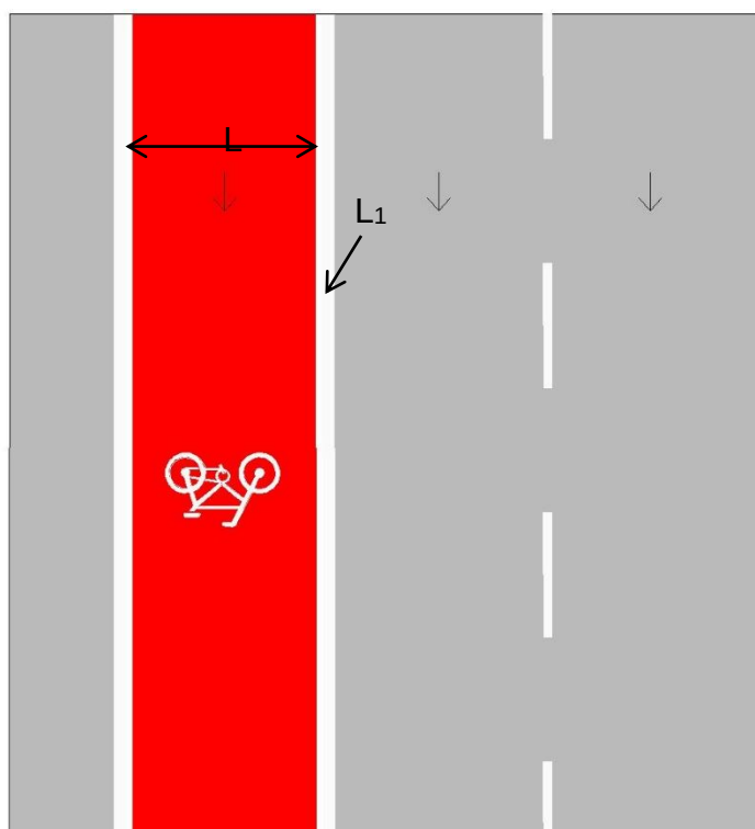
Figura 1: Marcação de ciclovia com superfície totalmente vermelha
