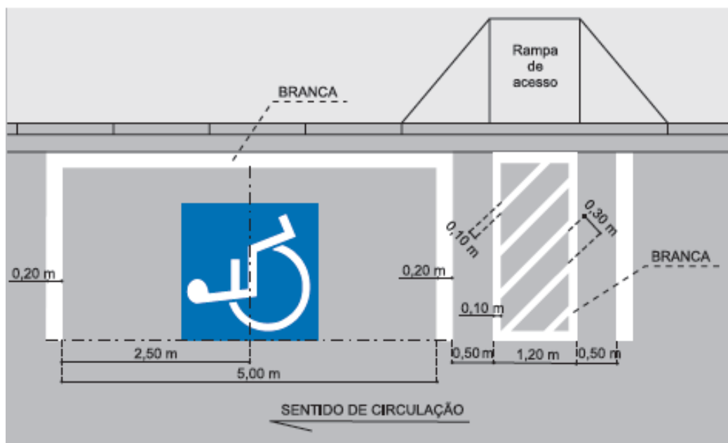
Figura 7: Detalhe de vagas de estacionamento destinadas exclusivamente a veículos que transportem pessoas portadoras de deficiência e com dificuldade de locomoção
