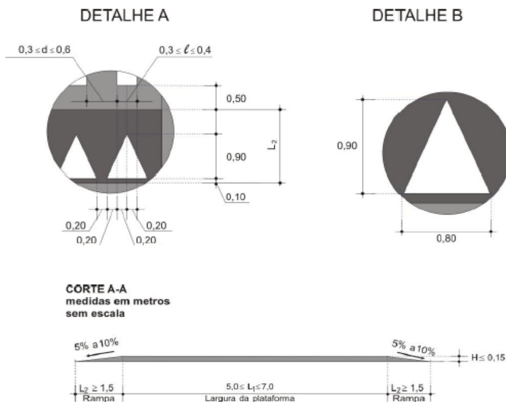
Figura 4: Detalhamento da faixa elevada
