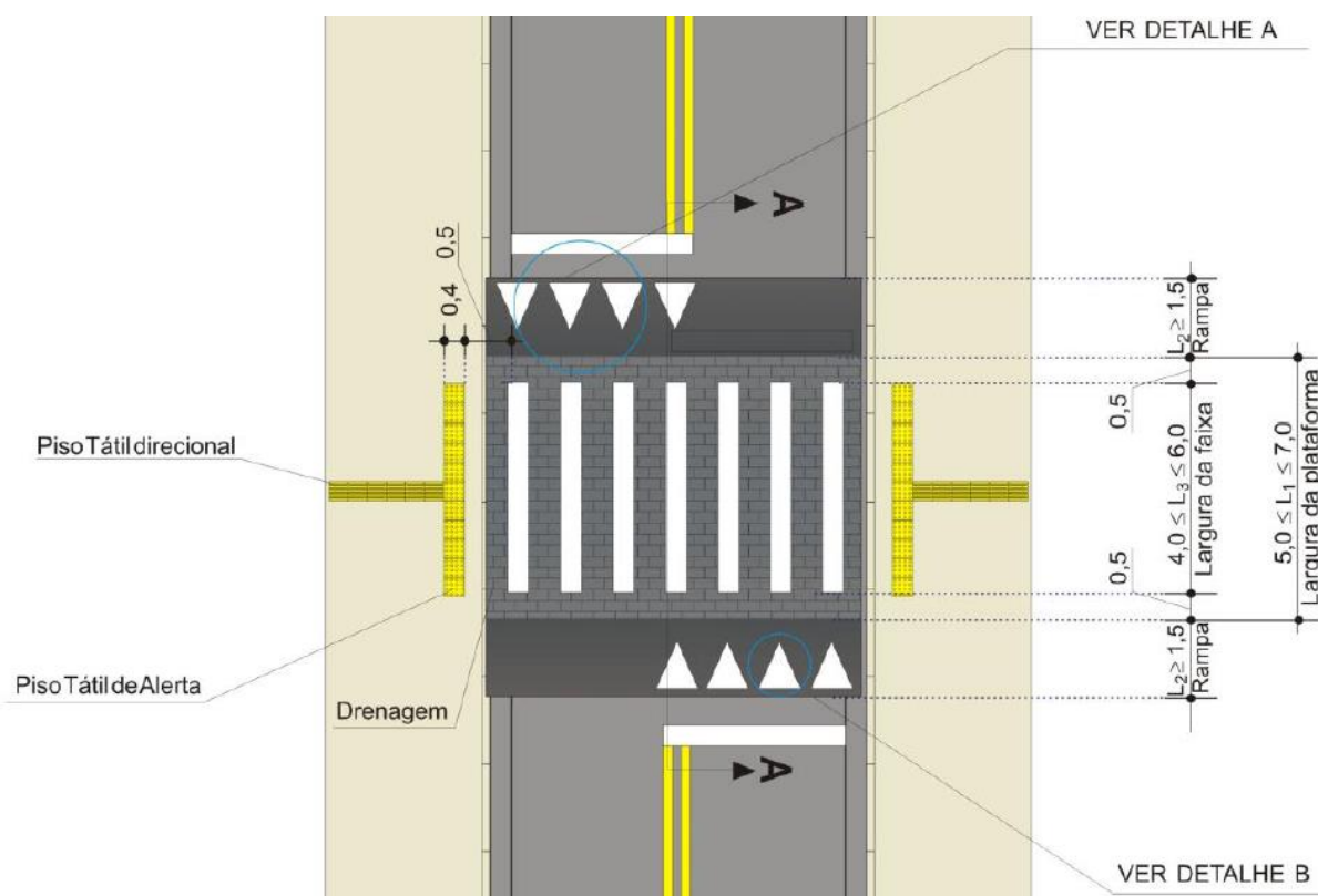
Figura 3: Visão geral da faixa elevada
