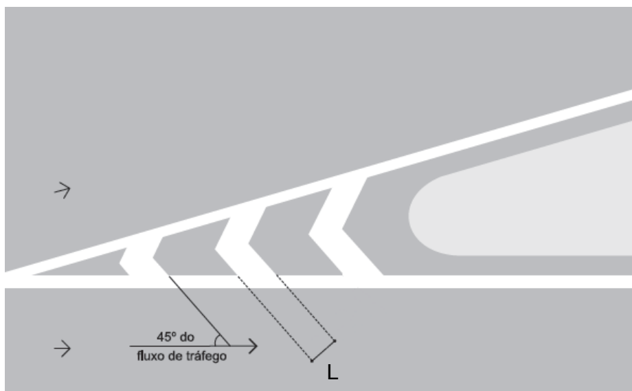
Figura 6: Detalhe de demarcação de ZPA
